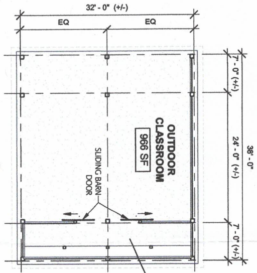
PLAN Scale: N.T.S.
